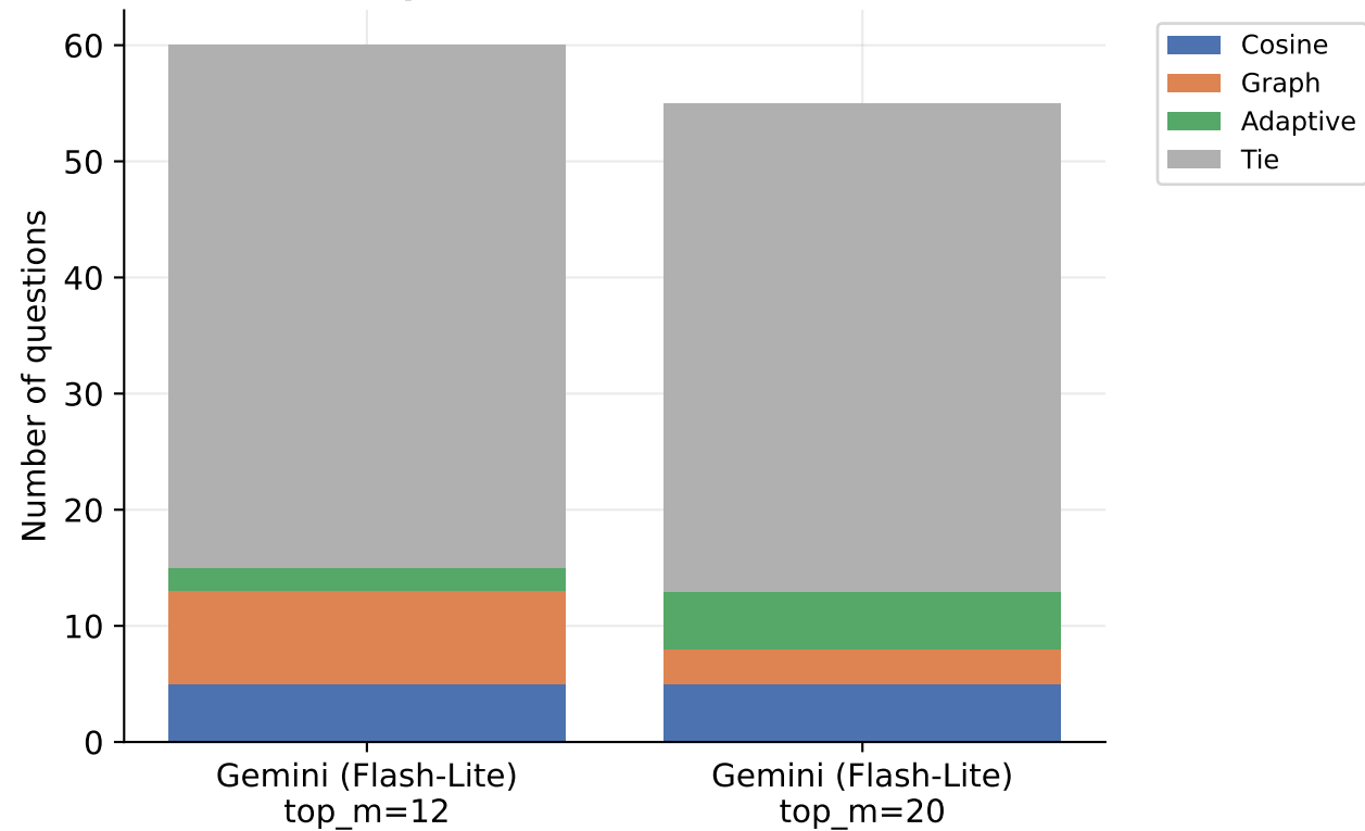
Per-question F1 winner - 2WIKI
